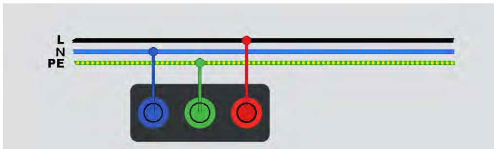
图 25. 用于接地电阻回路测试的 3 线连接（无跳闸模式）
