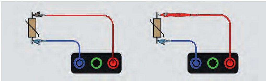
图 22. 压降测试连接
