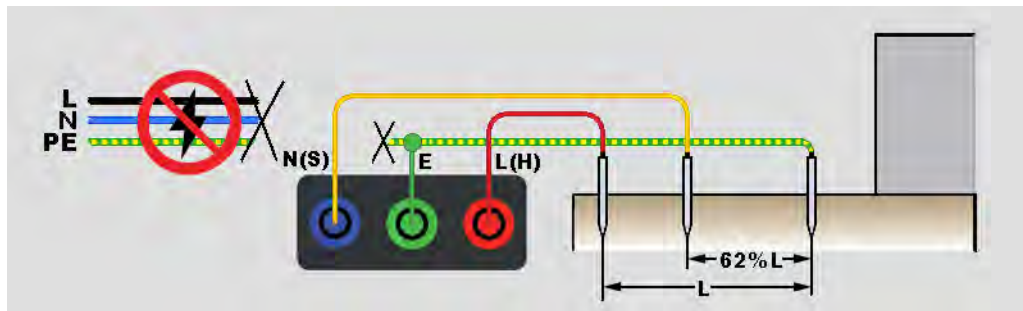
图 21. 接地电阻测试连接
