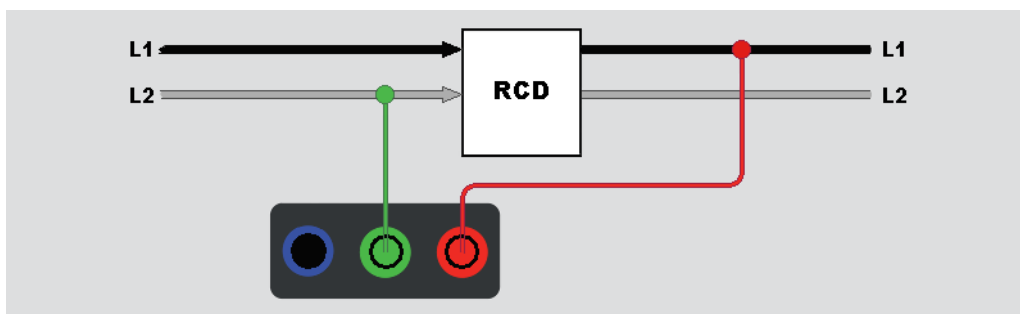
图 17. 用于在 IT 电气系统上进行 RCD 测试的连接
