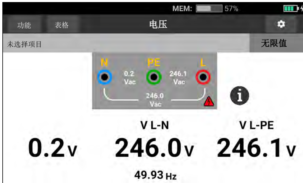
图 8. 电压和频率测量屏幕
