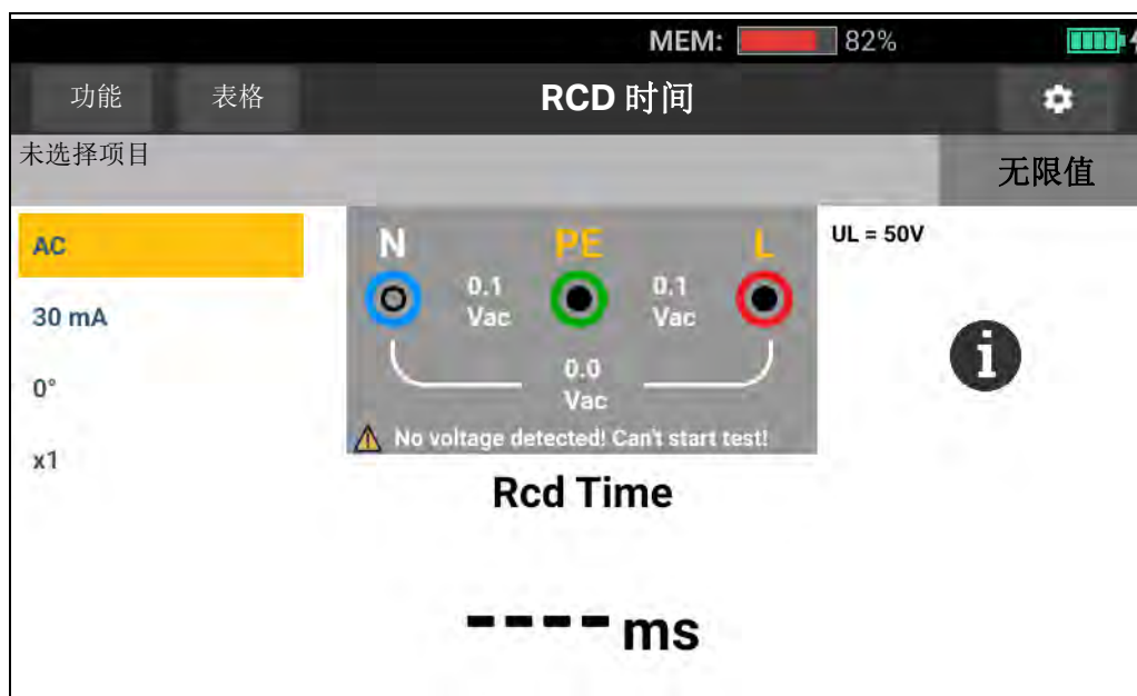
图 15.RCD 跳闸时间测量屏幕
