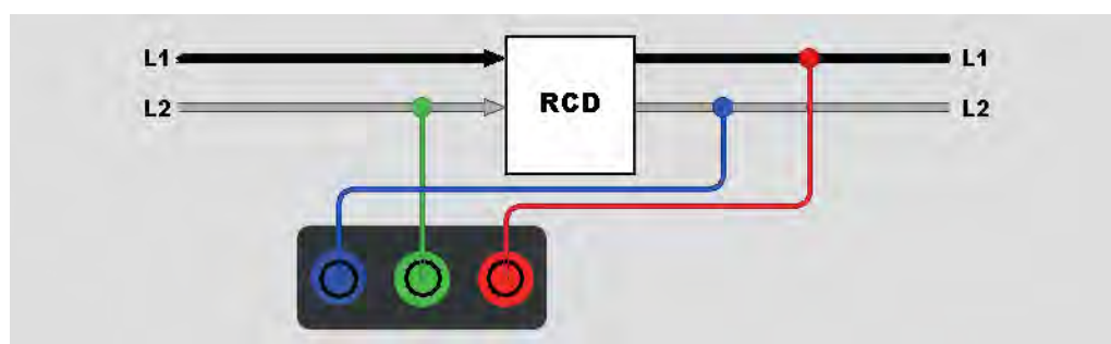
图 18. 用于在 IT 电气系统上测试 B 型 RCD 或 A-EV 型 RCD 的连接
