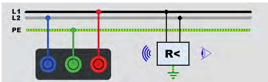
图 24.IMD 测试 #1
