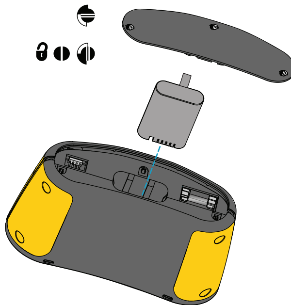
图 30. 电池更换
