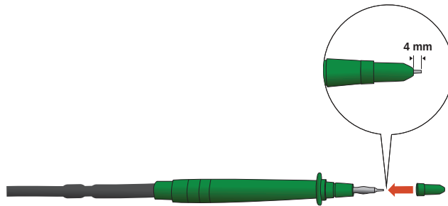
图 4. 带保护盖的测试导线
