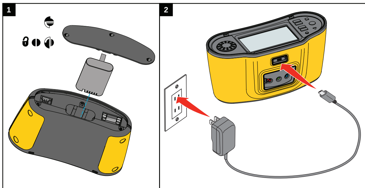
图 1. 使用 USB 电源为电池充电
