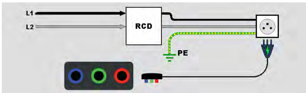
图 19. 单根测试导线配置
