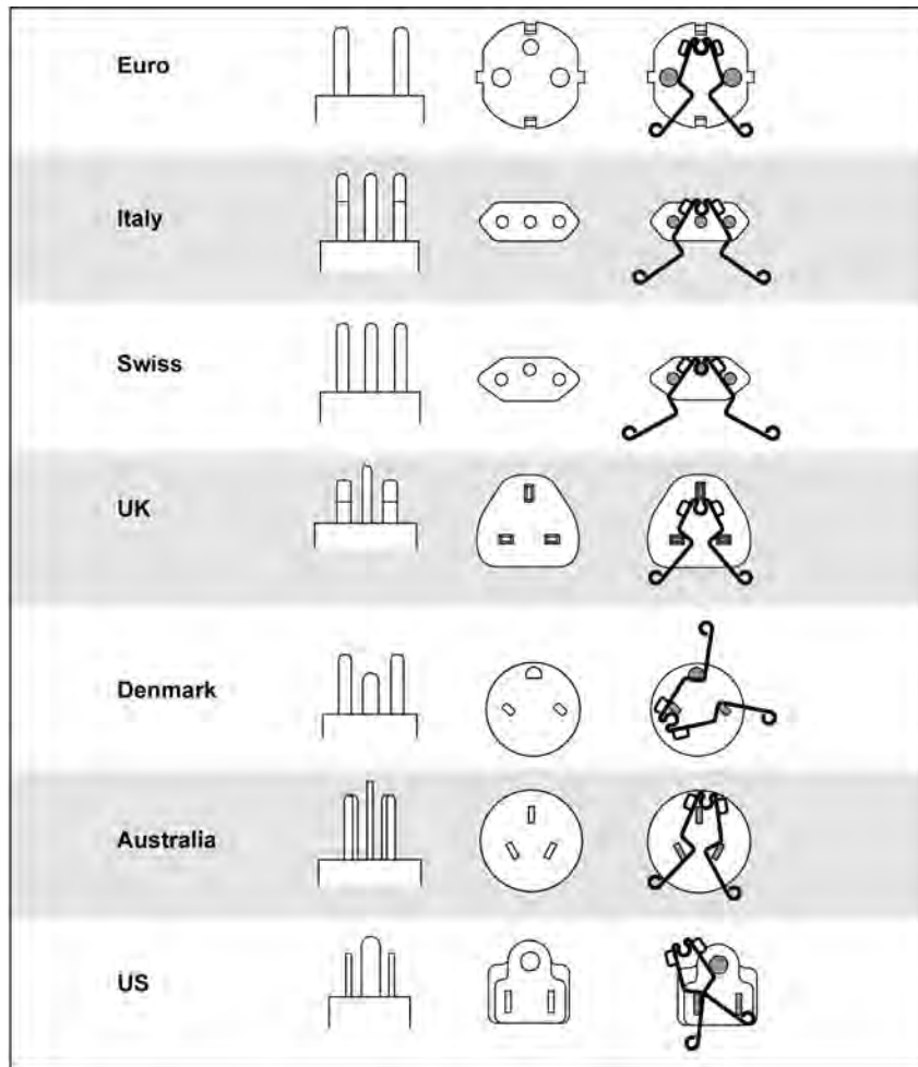
图 5. 特定国家 / 地区的调零适配器配置
