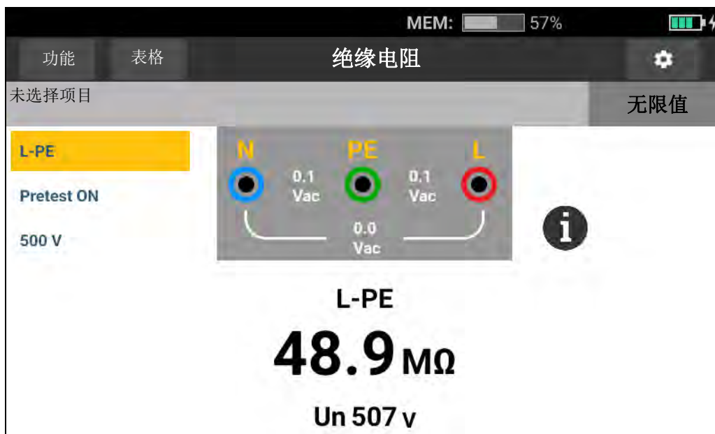
图 9. 绝缘电阻测量屏幕
