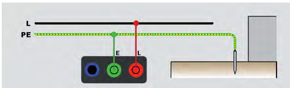
图 26. 用于接地电阻回路测试的 2 线连接（大电流跳闸模式）
