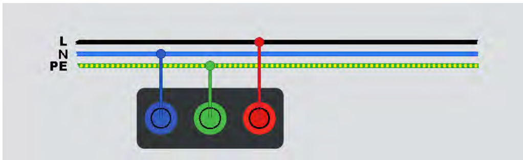
图 7. 安全预测试连接
