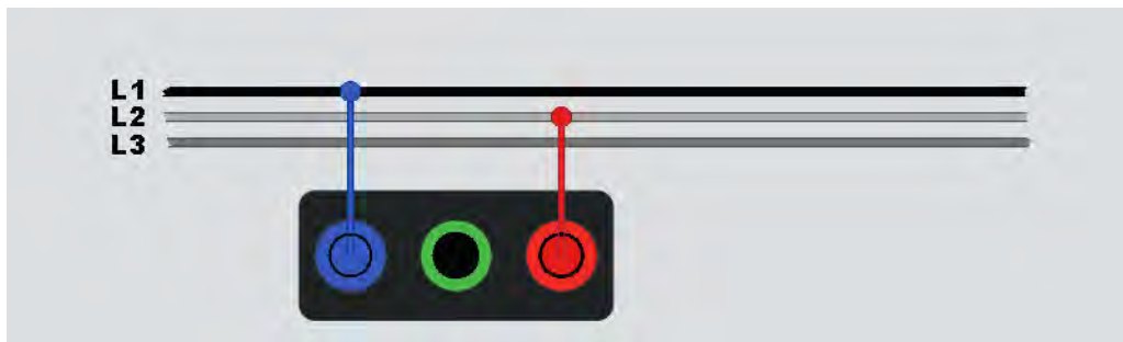
图 14. 三相系统测量
