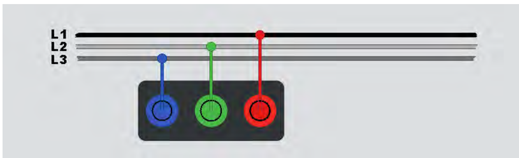
图 20. 相位旋转测试连接
